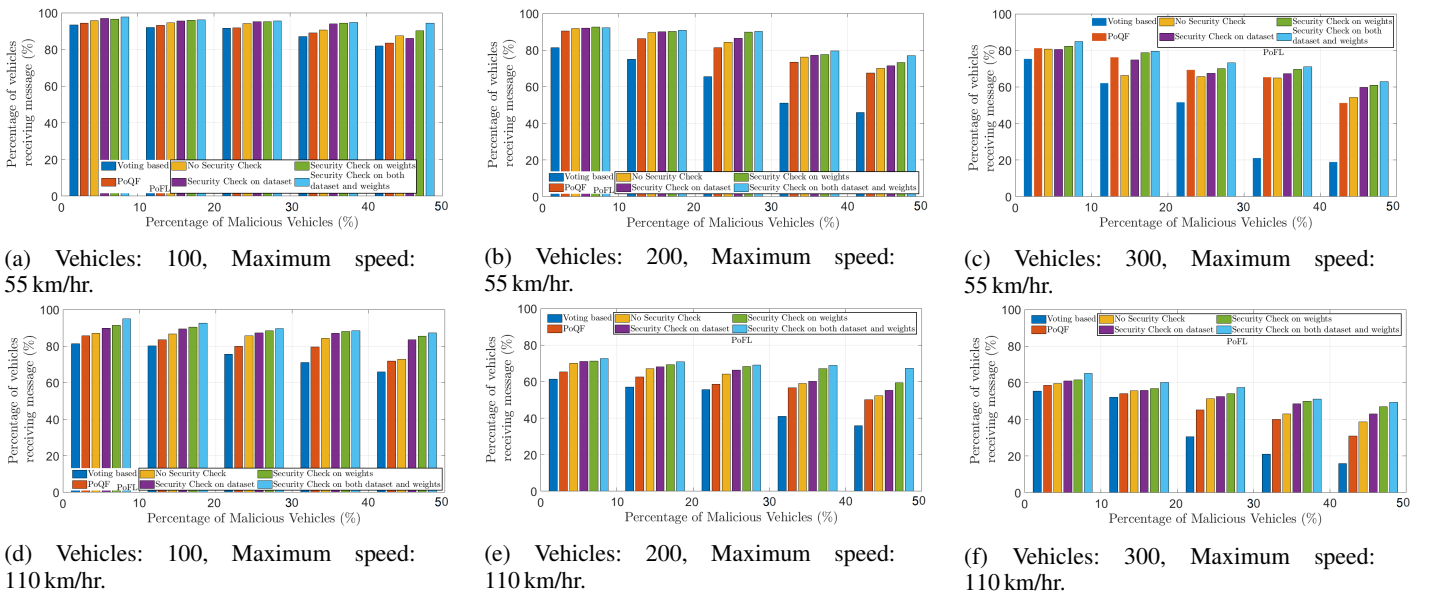
Fig. 12: Message delivery ratio.
