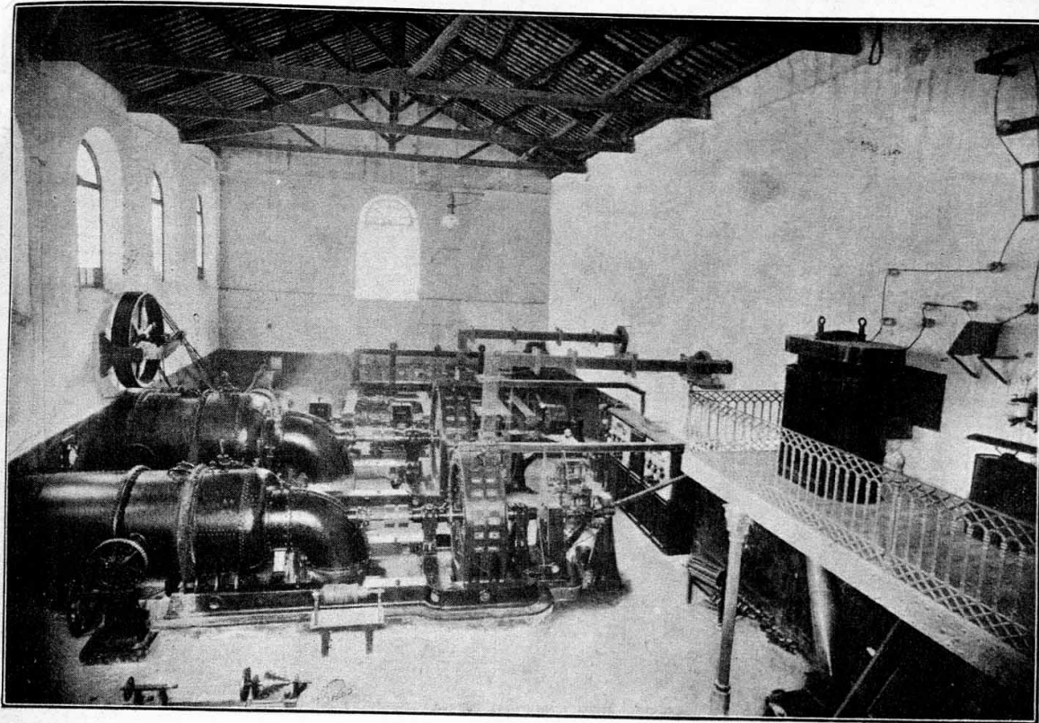
Gran estación electrógena para la alimentación de los hornos de carburo de calcio, manufactura agregada a las grandes industrias Sedó
