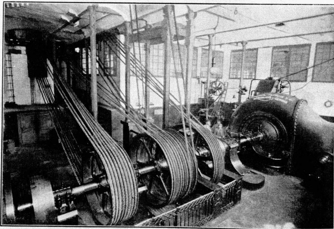
Gran sala de turbinas para la fuerza de las fábricas de hilados y tejidos
